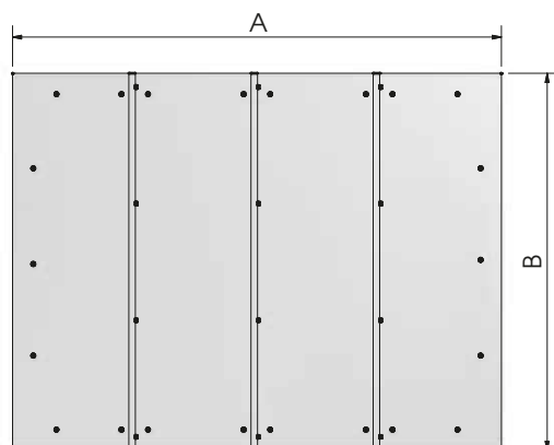
HRU-EC (dimensioni in mm)
