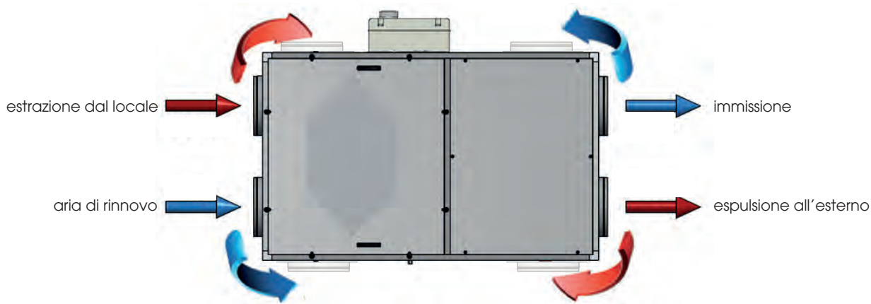
FAI-ED H (orizzontale) - VISTA DALL'ALTO
