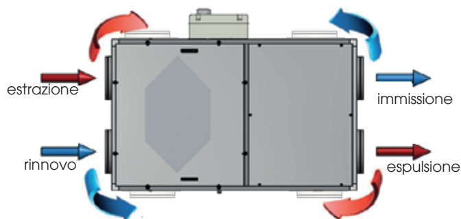
FAI-ED H (orizzontale) - VISTA DALL'ALTO
