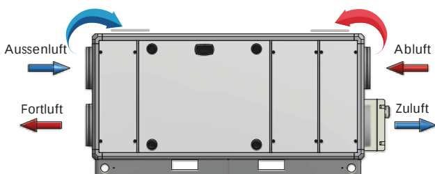
CRHE-V Seitenansicht
