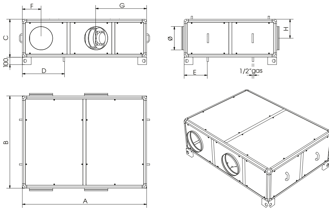
DIMENSIONI (mm) e PESI (kg)
