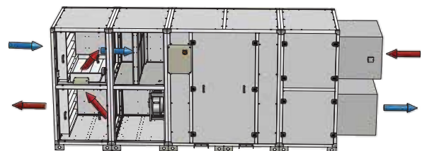
MODULE DE RECIRCULATION OUVERT
