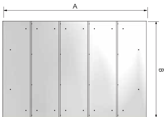
CRHE-V (dimensions en mm)
