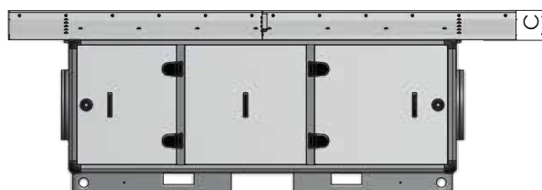
HRE-TOP EC (dimensions en mm)
