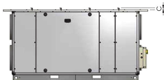
CRHE-V (dimensions en mm)
