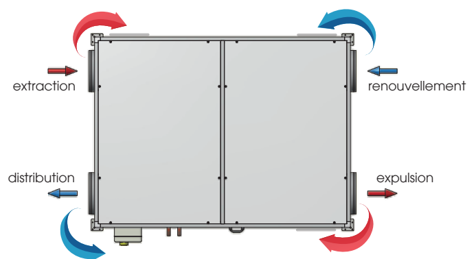
CRHE-H (horizontal) mirrored - VUE DU HAUT
