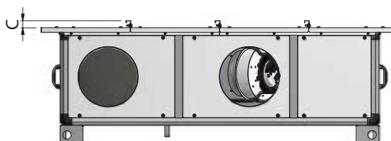
HRU-EC Abmessungen (mm)
