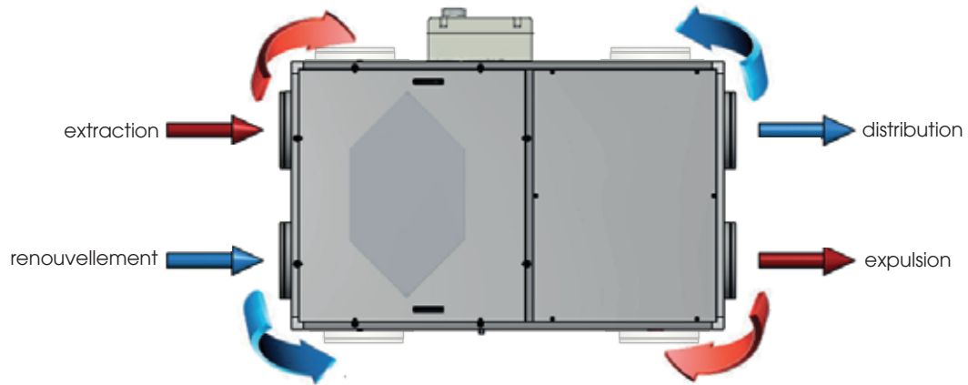
FAI-EC H (horizontal) - VUE DU HAUT
