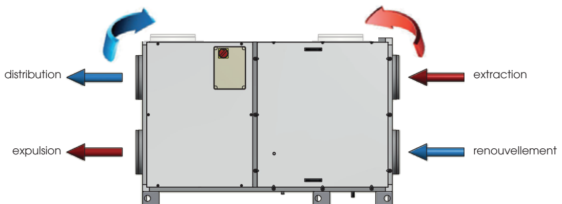
FAI-EC V (vertical) - VUE LATÉRALE
