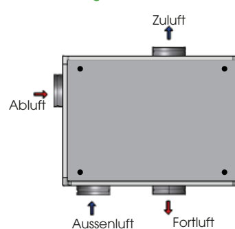
Konfiguration 2 miroir
