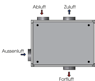
Konfiguration 3 miroir
