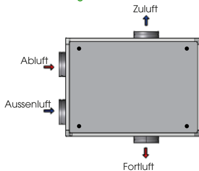
Konfiguration 4 miroir
