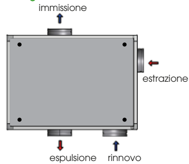
Configurazione 2 Standard
