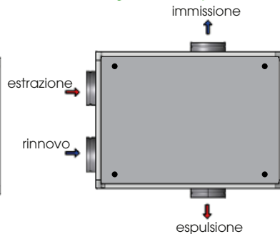
Configurazione 4 Specchiata
