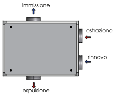
Configurazione 3 Specchiata
